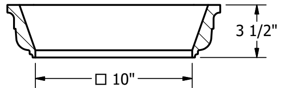
SECTION A-A
